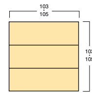
構造用管柱(S・P・F) 3ply
