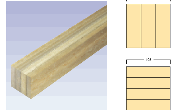
防腐防蟻処理土台(AQ認証)
